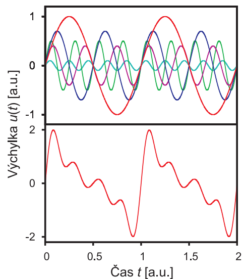
Obr. I.2.1 : Obrázek ukazuje časový vývoj výchylky u(x, t) v daném bodě x , kterým prostupuje 5 harmonických vln 1 \sin \varphi , 0,7 \sin 2\varphi , 0,4 \sin 3\varphi , 0,5 \sin 4\varphi a 0,1 \sin 5\varphi , kde \varphi = \omega(t - x/c) . Jednotlivé harmonické kmity odpovídající vlnám jsou zobrazeny na obrázku nahoře a výsledné kmitání na obrázku dole. Perioda (a tím i frekvence) výsledného kmitání odpovídá periodě kmitů vlny s nejnižší frekvencí f_1 = \omega/2\pi .
