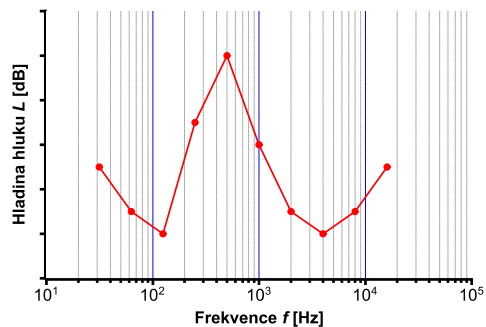
Obr. I.2.5 : Příklad zjištěné frekvenční závislosti hladiny hluku. Zde je výrazné maximum okolo frekvence 500 Hz. Bude-li zdroj hluku odstraněn či utlumen jeho ak. výkon, poklesne i celková hladina hluku.
