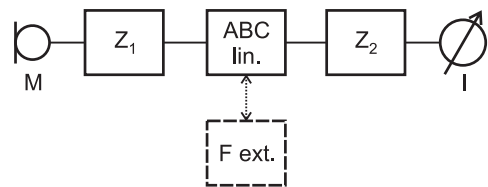
Obr. I.2.4 : Blokové schéma zvukoměru.
